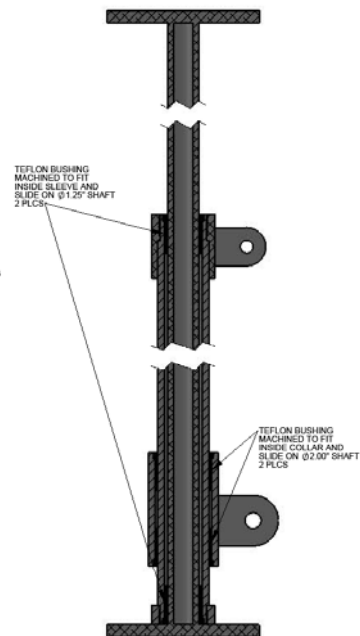
SECTION D-D SCALE 1 : 2
